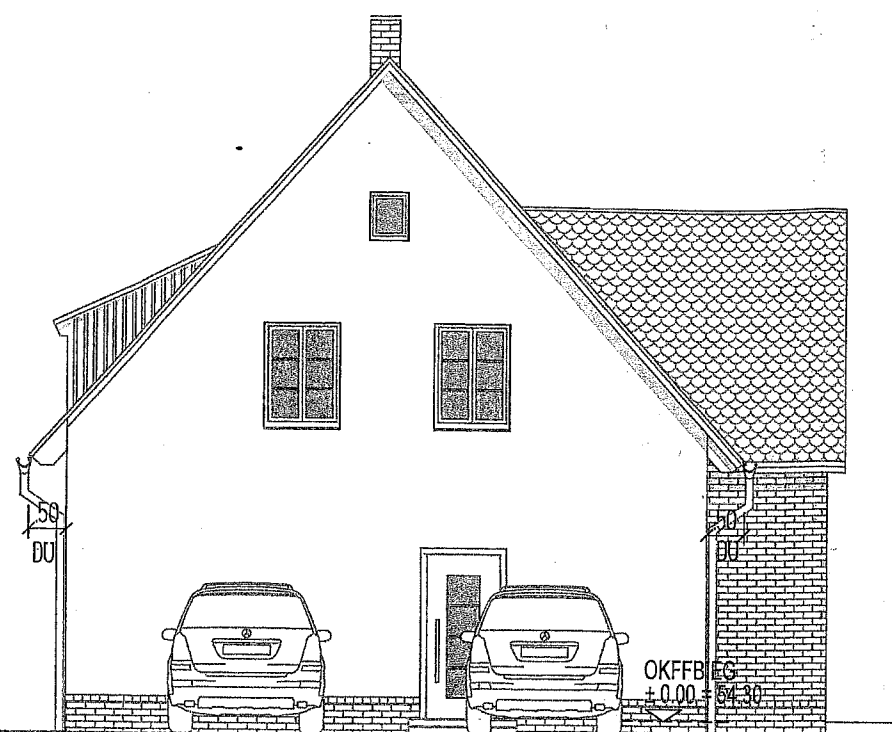
ANSICHT SÜDWEST
