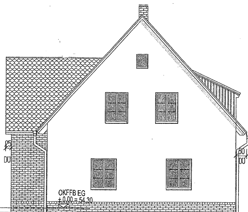
ANSICHT NORDOST
